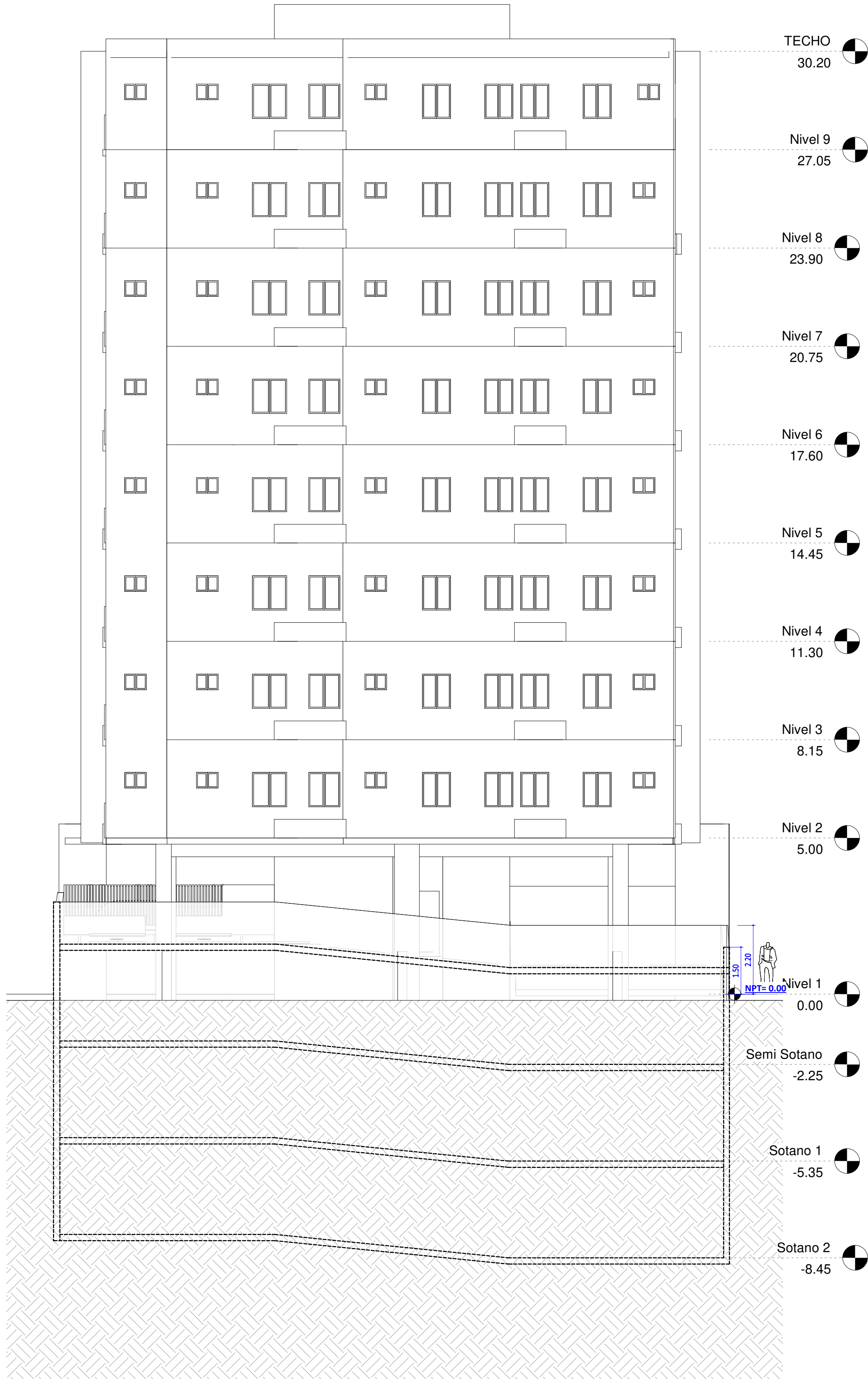
ELEVACION POSTERIOR (03)
