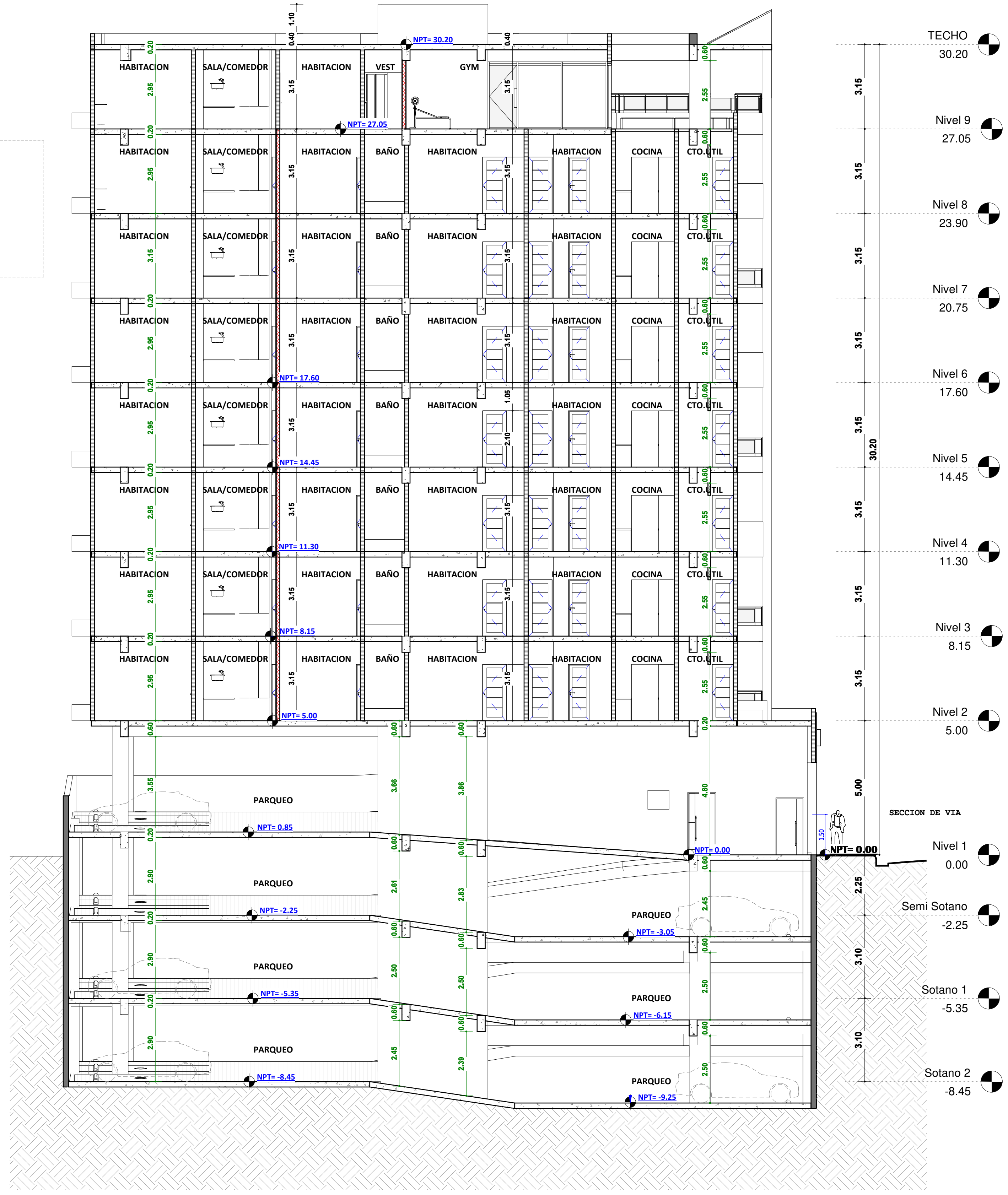
SECCION LONGITUDINAL (L1)
