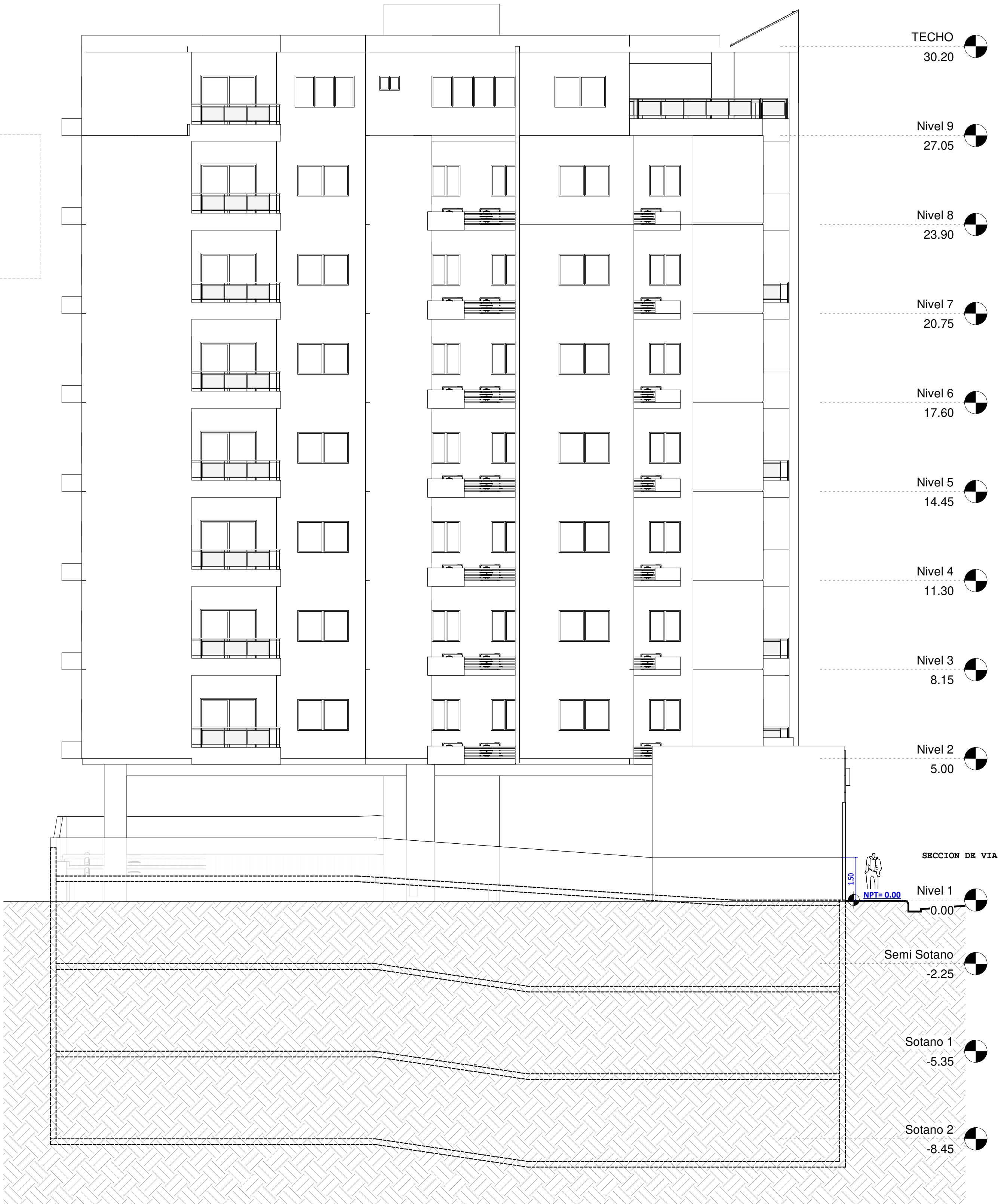
ELEVACION LATERAL IZQUIERDA (04)
